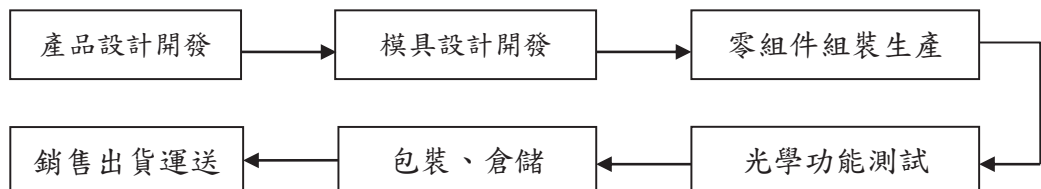
光纖連接器生產作業流程
